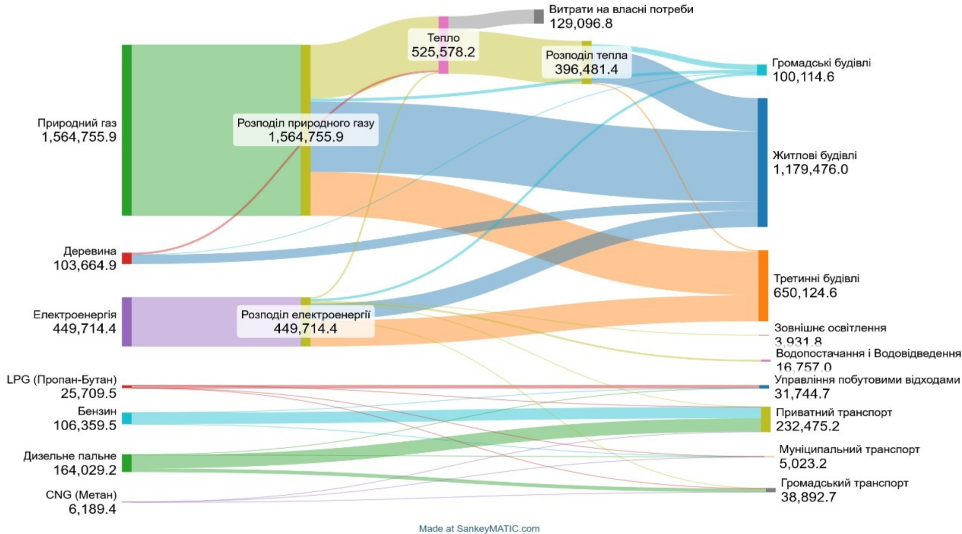
На рисунку 2.15 Діаграма Sankey у графічному вигляді відображено енергоспоживання в Луцькій МТГ на 2024 рік
