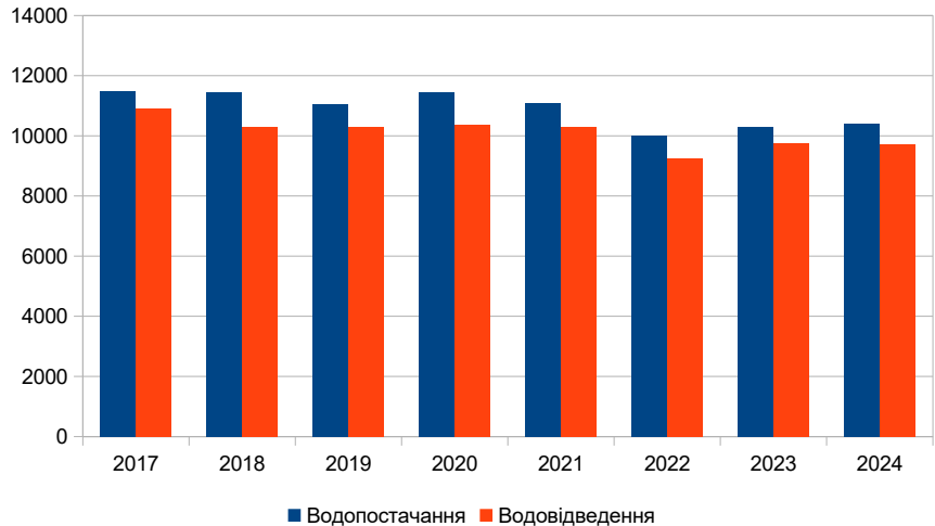
Рисунок Д2.10. Динаміка обсягів водопостачання та водовідведення, тис.м³ Загальна кількість абонентів з водопостачання та водовідведення приведена у таблиці Д2.14. та на рисунку Д2.11. Відсоток абонентів, що мають встановлені прилади обліку поступово зростає і на 2025 рік складає 91,99 % від усіх абонентів. Враховуючи постійний ріст тарифів на водопостачання та водовідведення відсоток встановлених лічильників буде зростати та наближатися до відмітки 100 %.
