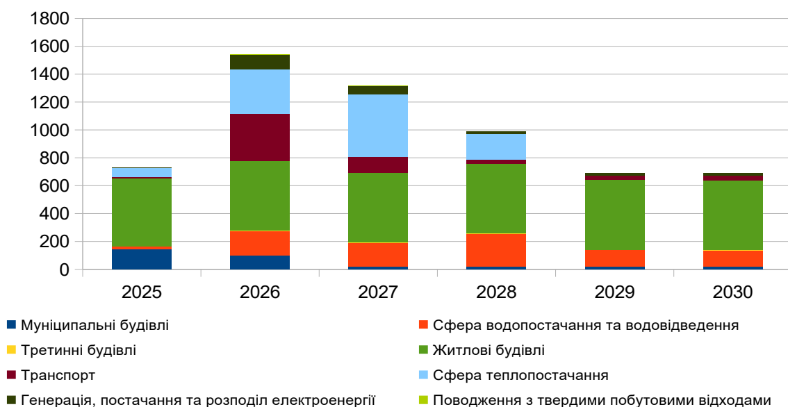
Рисунок 5.1. Зведений інвестиційний баланс за категоріями кінцевих споживачів
