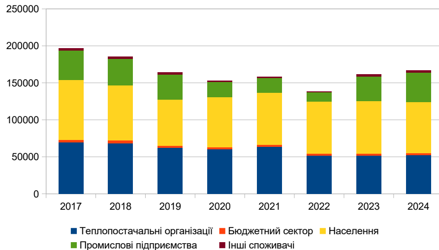
Рисунок Д2.22. Споживання природного газу споживачами, тис.м 3
