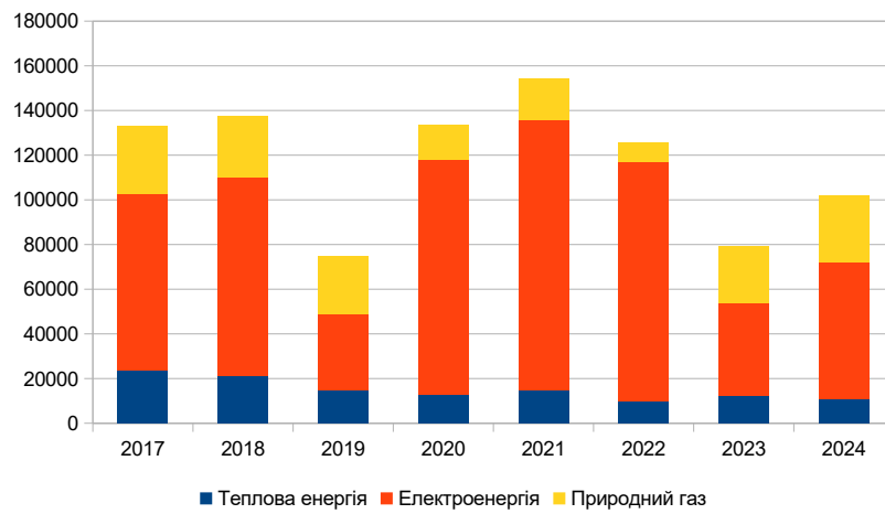
Рисунок Д2.25. Споживання енергоресурсів промисловістю та комерційними структурами, МВт.год
