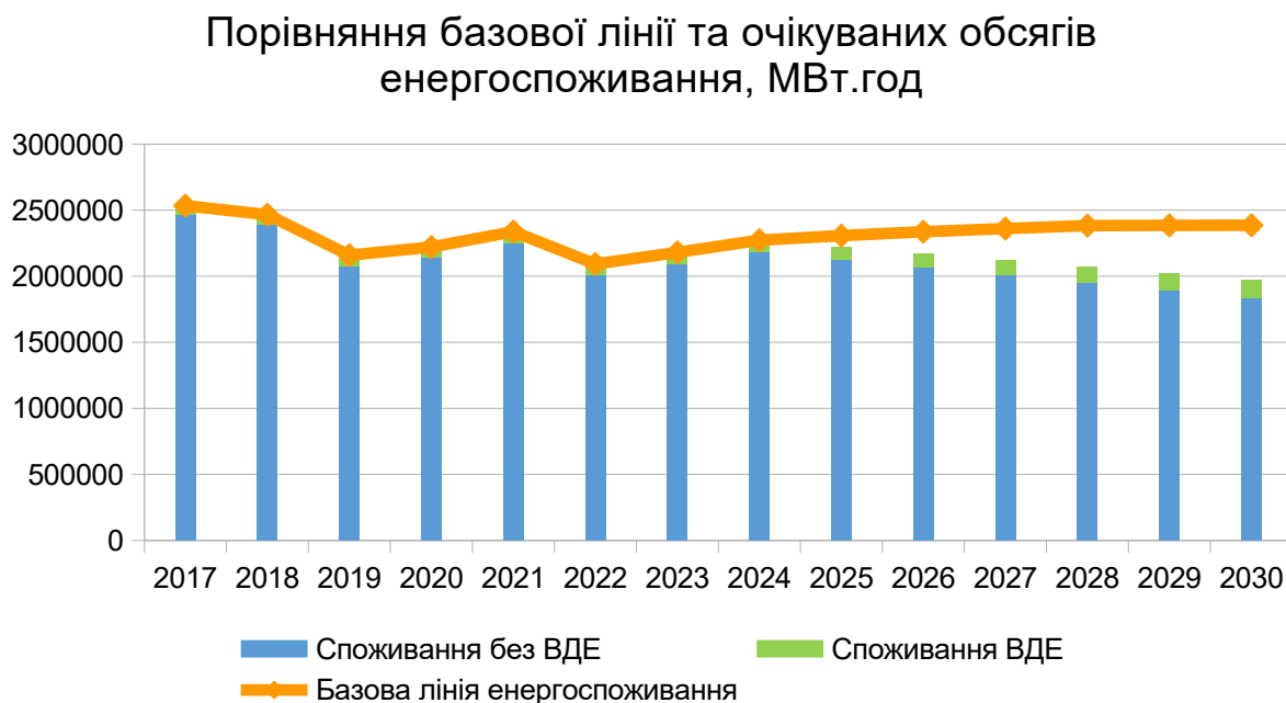
Рисунок 3.1 Базова лінія споживання енергії в Луцькій МТГ
