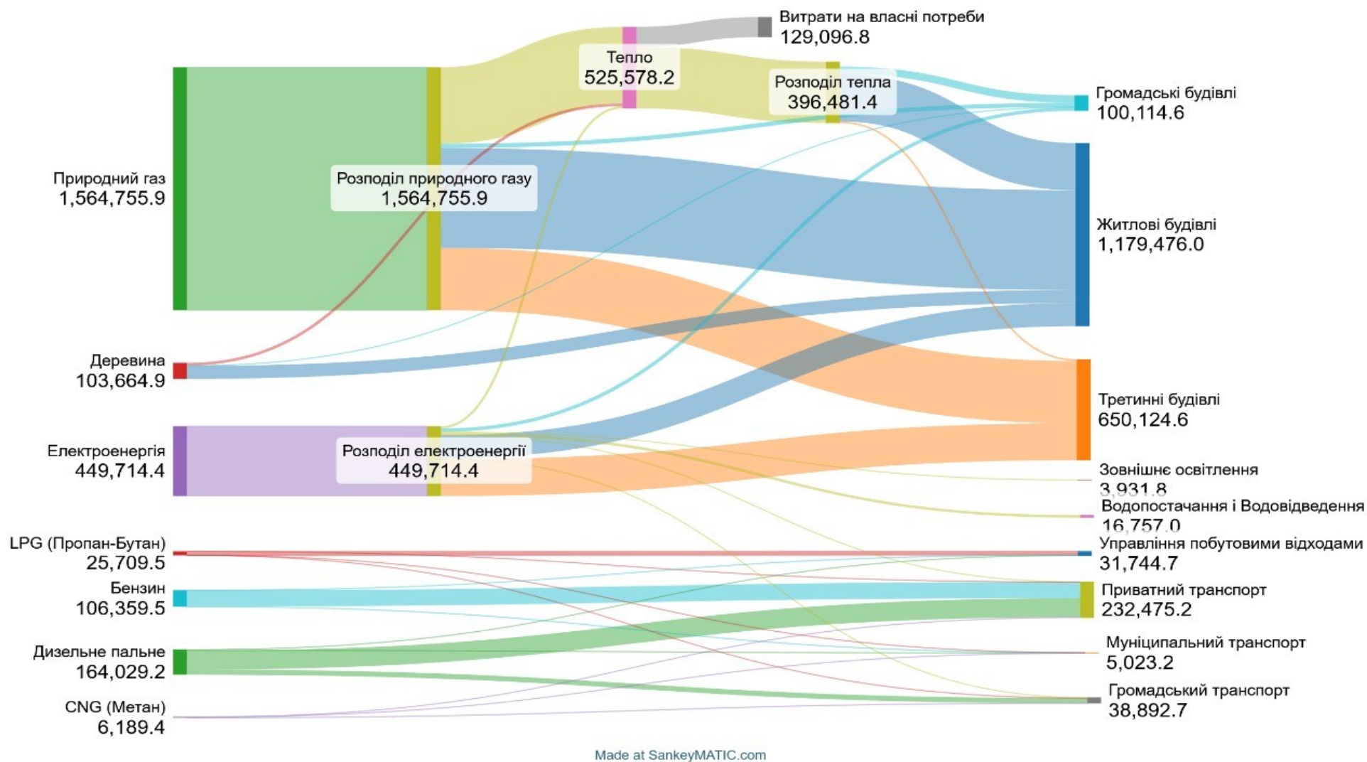
Рисунок 2.15. Діаграма Sankey енергетичного балансу Луцької МТГ за 2024 рік, МВт·год
