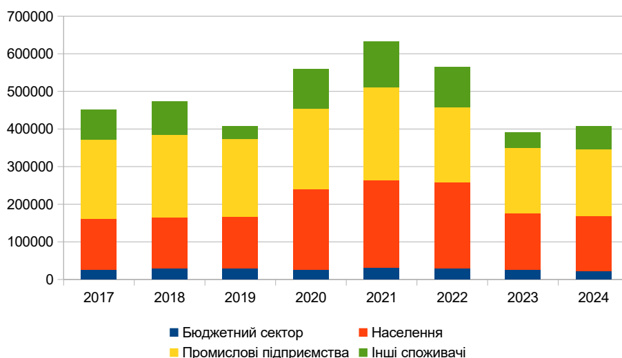
Рисунок 2.10. Обсяги постачання електроенергії споживачам Луцької МТГ, МВт·год
