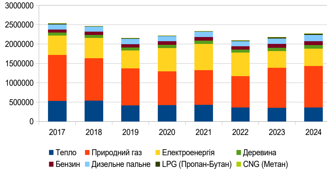
Рисунок 2.17. Зведений енергетичний баланс за видами енергії, МВт·год
