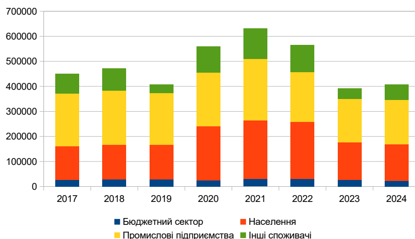
Рисунок Д2.23. Обсяги постачання електроенергії споживачам Луцької МТГ, МВт.год Між 2017 та 2021 роками спостерігається зростання споживання електричної енергії на 40 % (рис. Д2.23.). Однак, у 2022-2024 роках відбувся спад причиною якого є пошкодження інфраструктури в результаті воєнних дій РФ проти України.
