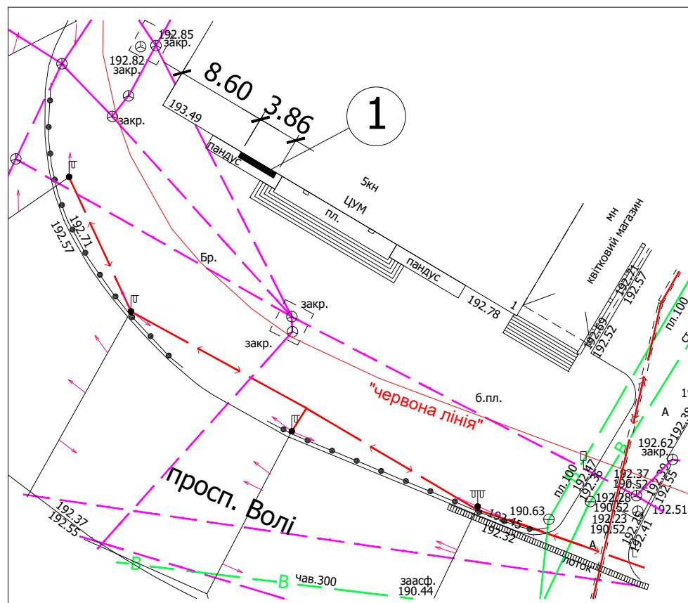
Схема розміщення засобу зовнішньої реклами, М 1:500
