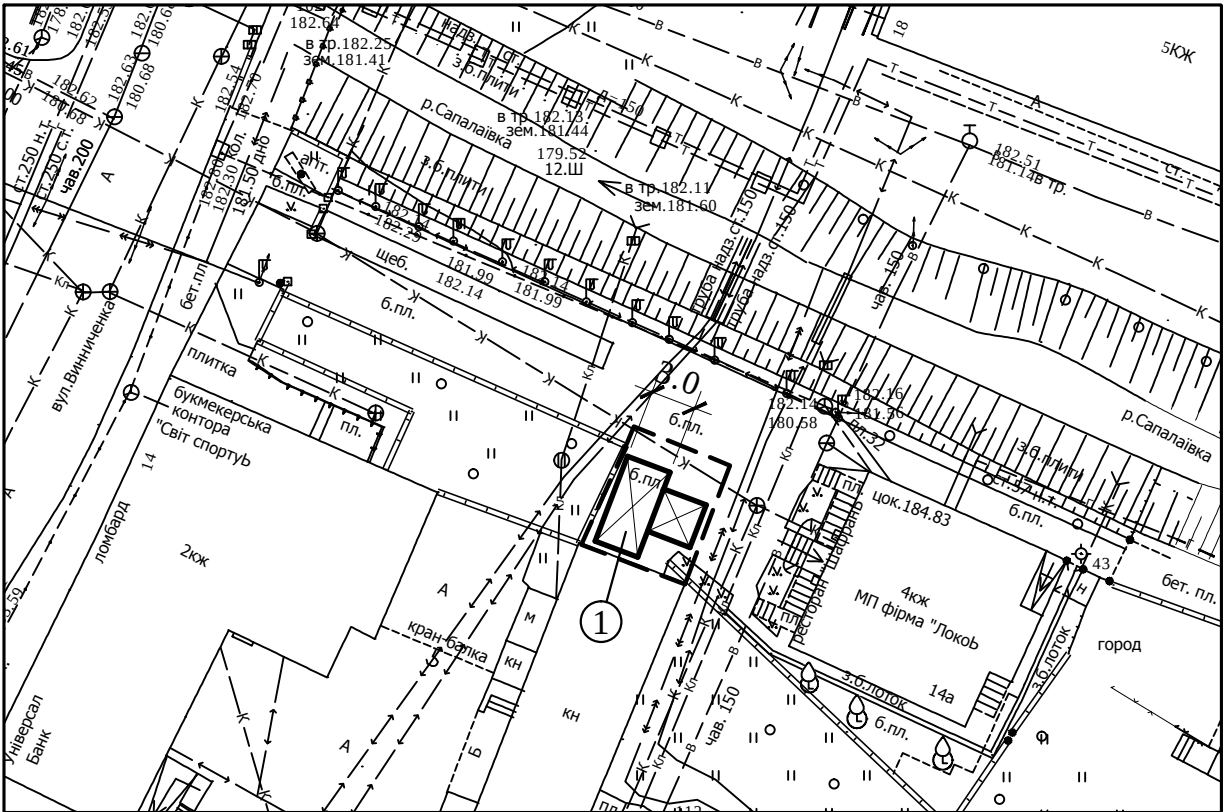
Схема розміщення тимчасової споруди, М 1:500
