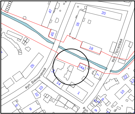
Схема розміщення тимчасової споруди, М 1:500
