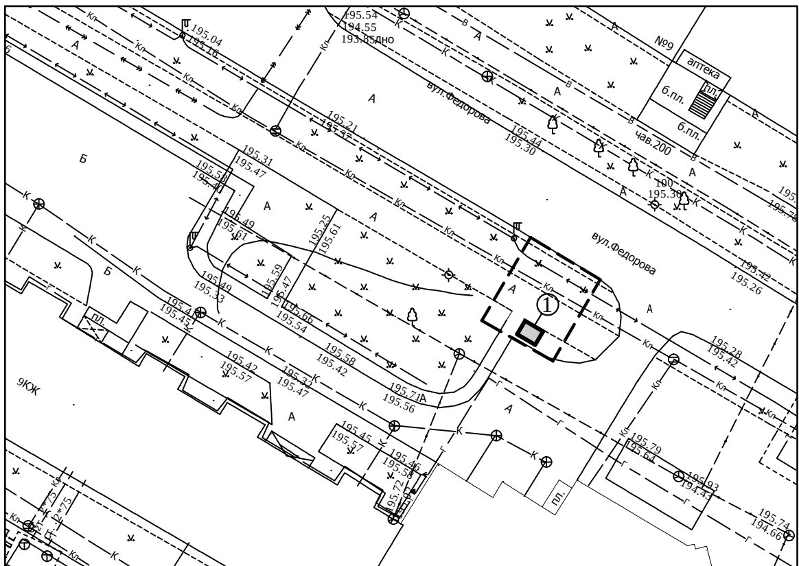
Схема розміщення тимчасової споруди, М 1:500
