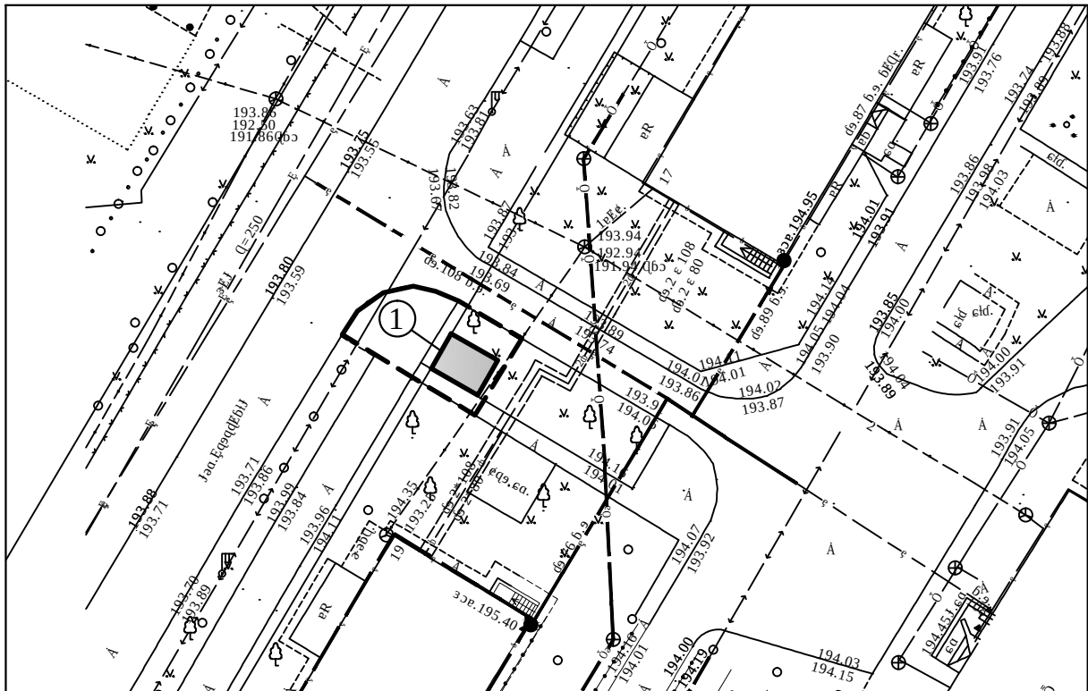
Схема розміщення тимчасової споруди, М 1:500
