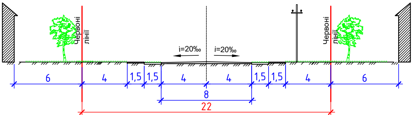
Поперечний профіль 1-1, М 1:200
