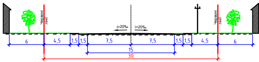
Поперечний профіль 1-1, М 1:200
