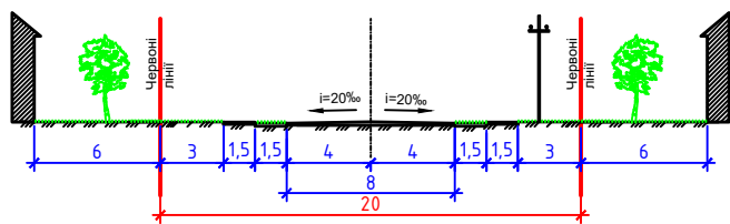
Поперечний профіль 2-2, М 1:200
