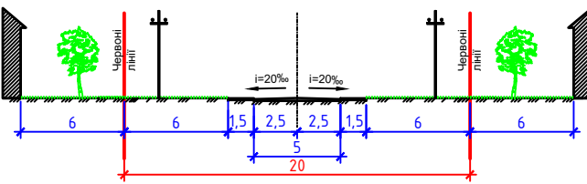
Поперечний профіль 1 - 1, М 1:200
